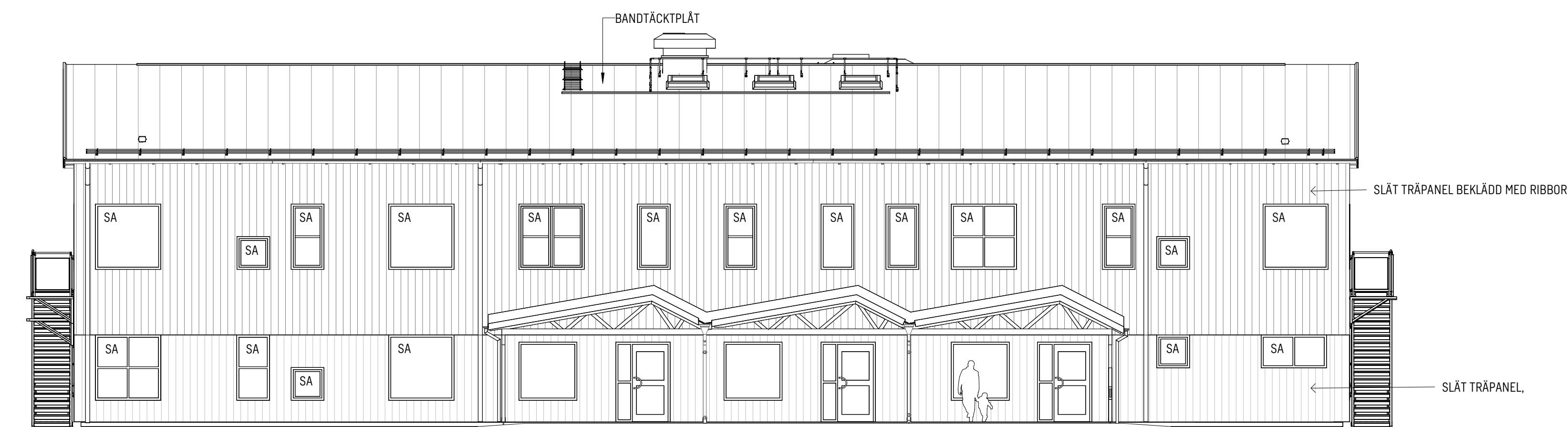
FASAD A (MOT GÅRD) 1 : 100
