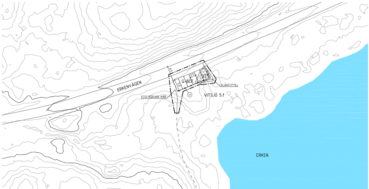
Bilaga 2. Ritning över de befintliga samt planerade parkeringsrutorna. Utökad yta = prickad yta i öster markerad med G1. G-BEF = befintlig grusyta där ingen ny åtgärd ska utföras.
