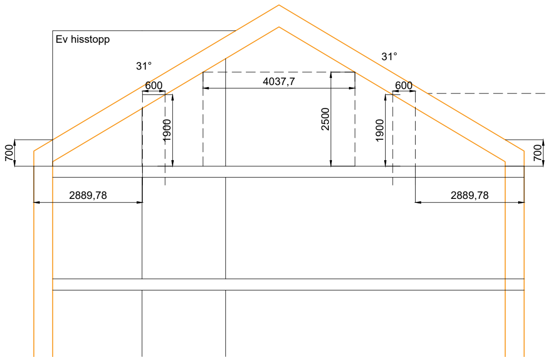
Ca 20 förråd / trapphus ihop med yta för fläktrum och trapphuset Skissen förhåller sig till gällande funktionskrav i komplementsutrymmen för bostäder och utgår från en vinkel på ca 30 graders tak i förhållande till typtrapphuset.
