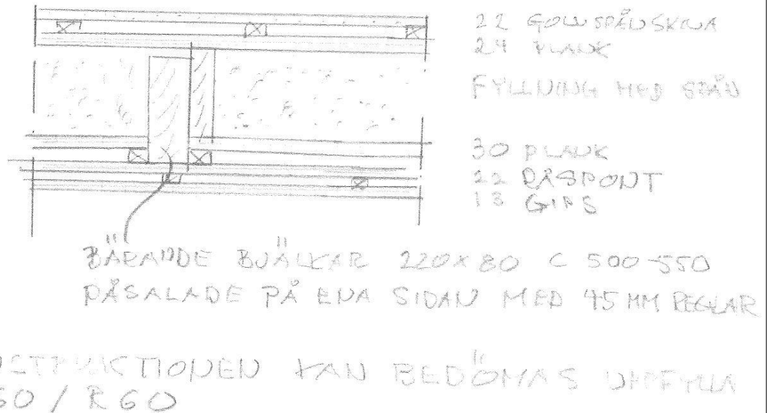
Figur 1. Bjälklag mellan butiker och bostäder. Källa: Brandskyddsdocumentation som relationshandling för Kv Venus 9.
