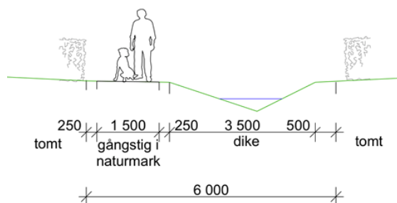
Figur 42 Principsektion av släpp mellan tomter för gångstig och dike.
